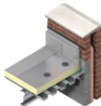
dach płaski - Therma
